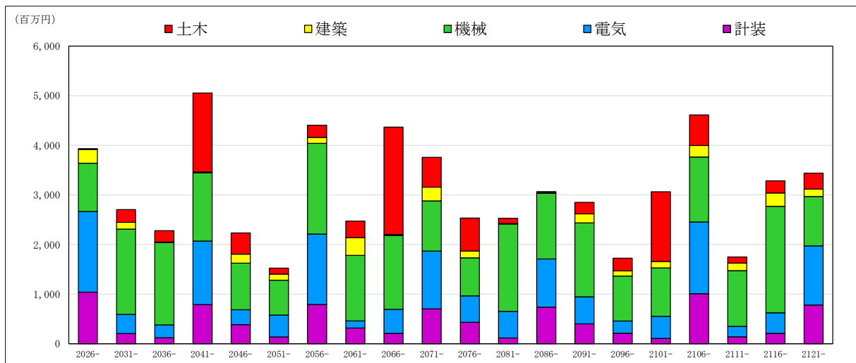
図 3.2.4 施設の更新需要（更新基準年数で更新）ケース②
