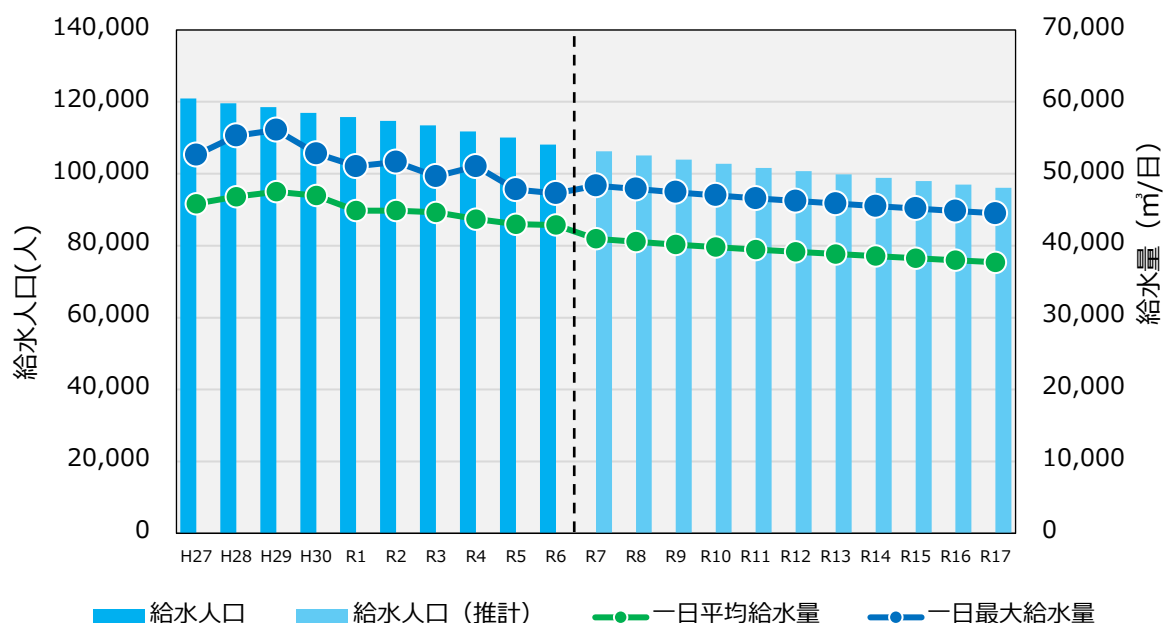
図 3.1.1 給水人口・給水量の見通し
