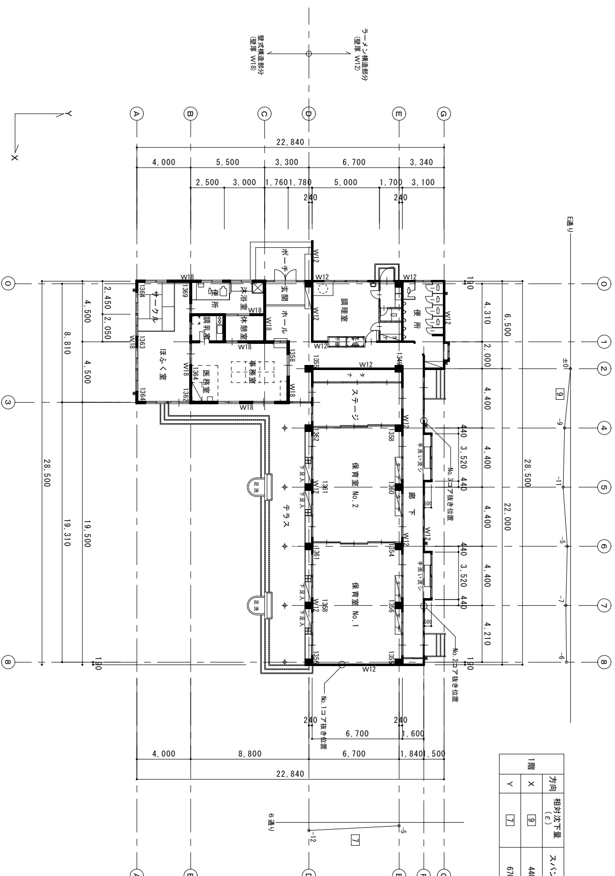
平面图 S=1:200
