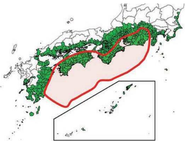
南海トラフ地震の想定震源域と南海トラフ地震防災対策 推進地域（内閣府資料に一部加筆）
