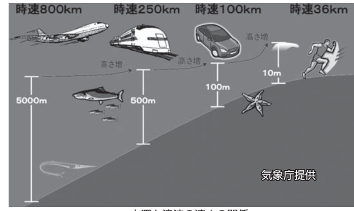
水深と津波の速さの関係
