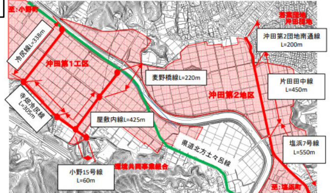
平面図
