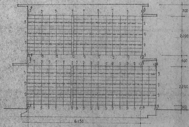
A通り ブロック割図
