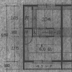
2階平面図 25.83 m
