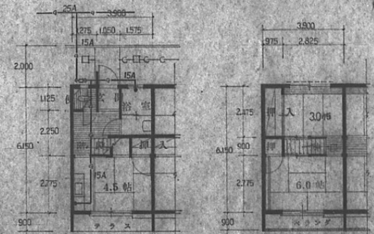
1階平面図 23.98 m
