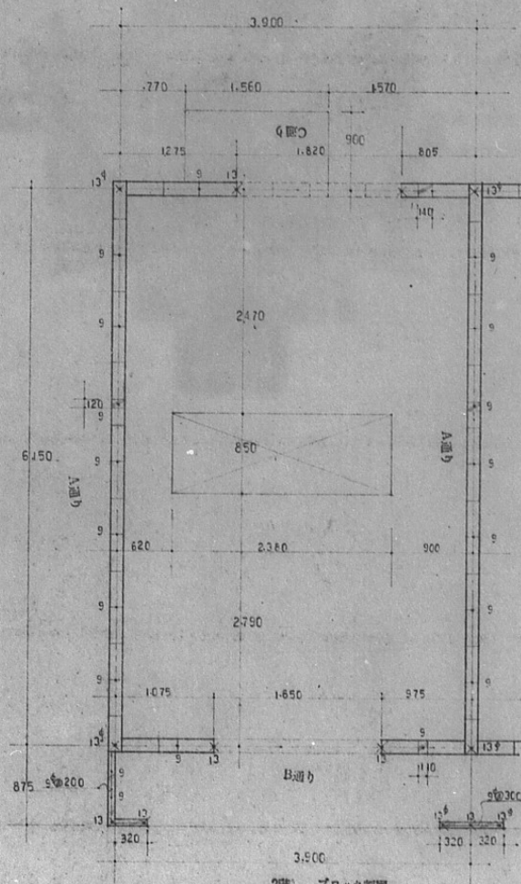
F通り ブロック割図
