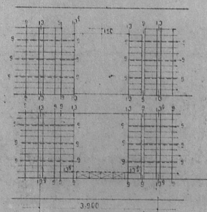
B通り ブロック割図
