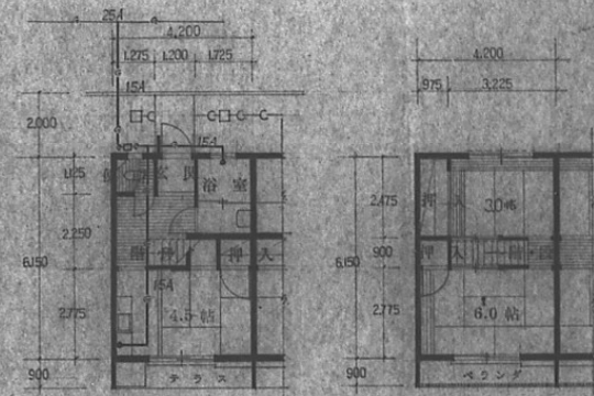
1階平面図 25.83 m
