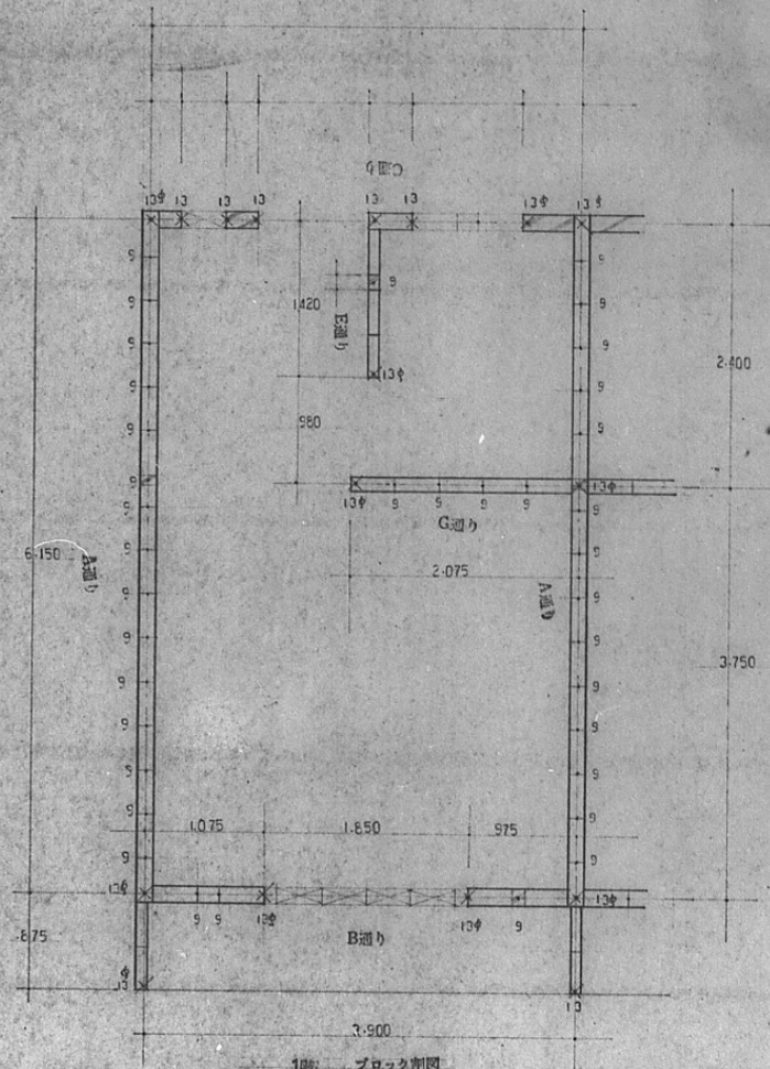
E通り ブロック割図
