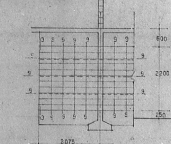
D通り ブロック割図
