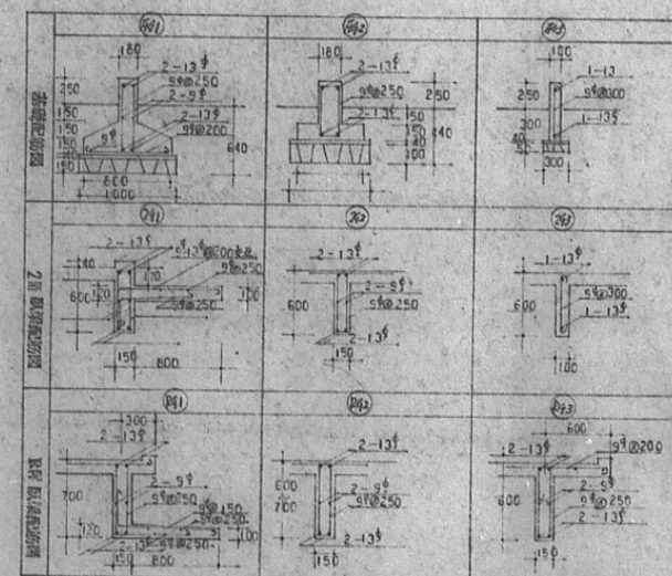
R階段断面図 S = 100
