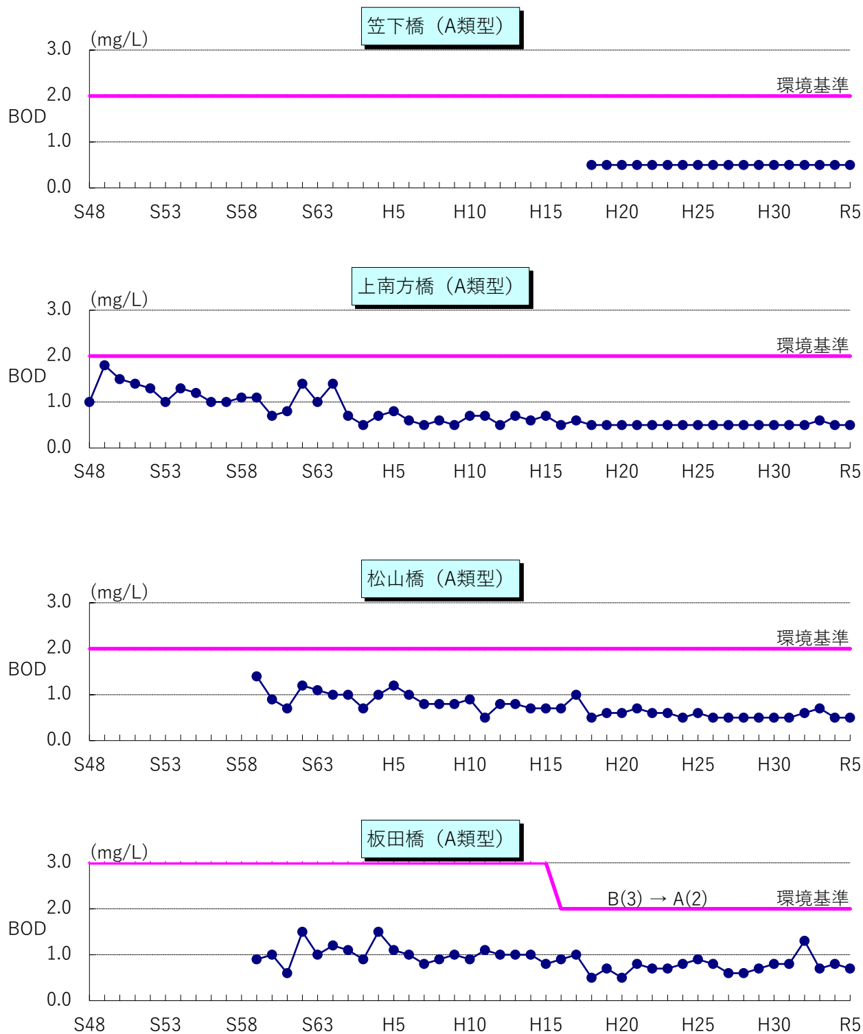
図25 五ヶ瀬川のBOD経年変化
