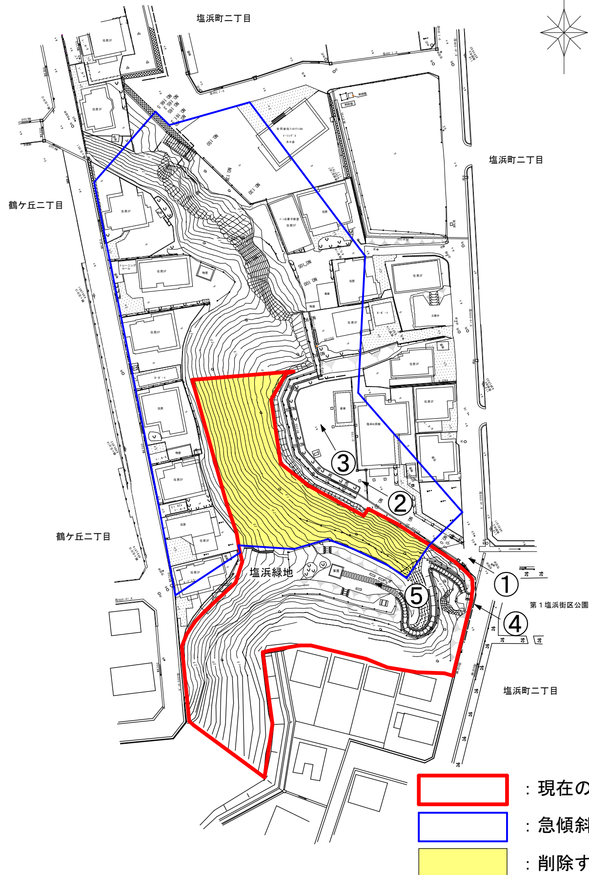
塩浜緑地 平面図 S=1/1000
