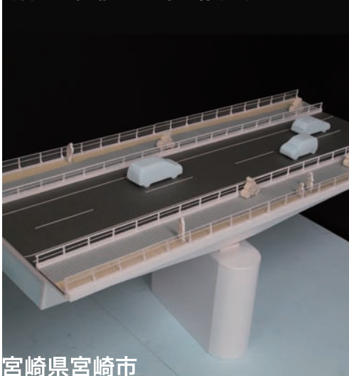
昭和通線橋上・街路景観デザイン
